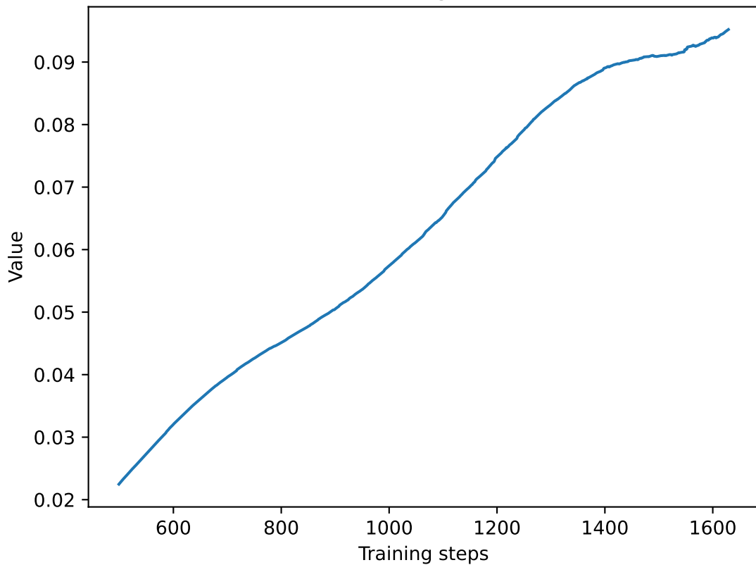
KL divergence
